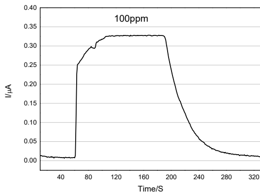
传感器灵敏度及响应恢复特性
