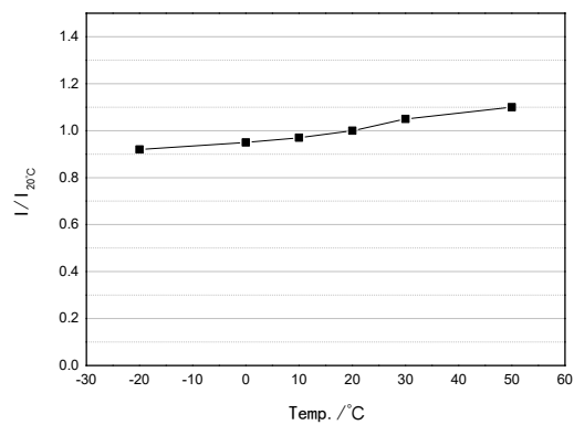
传感器不同温度下零点特性
