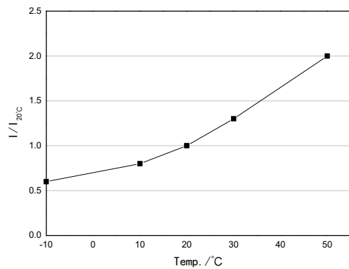
传感器不同温度下输出特性
